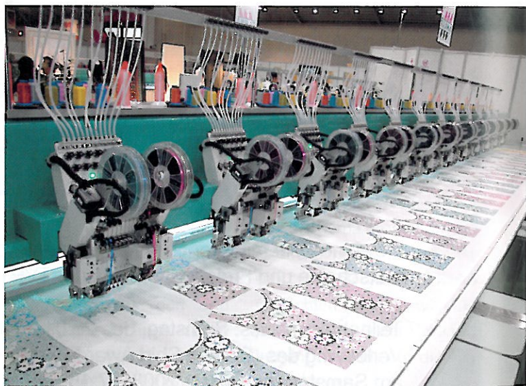
Die Tandem-Pailleteneinrichtung für die TFGN-Maschinen von Tajima
